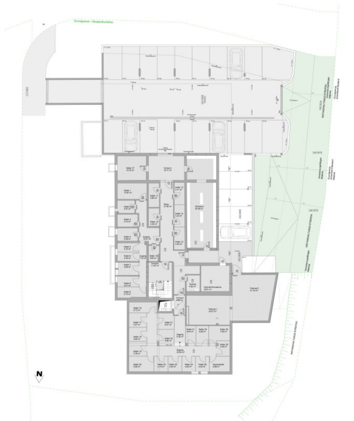
Grundriss Untergeschoss
