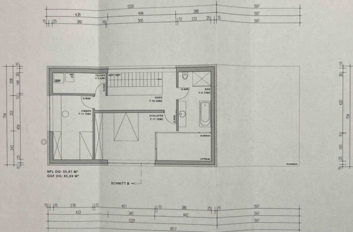
GRUNDRISS OBERGESCHOSS M1:100
