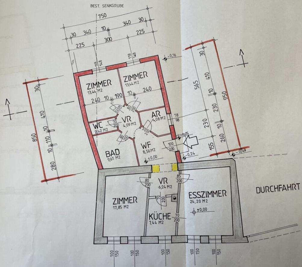
GRUNDRISS
