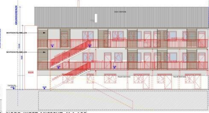
NORD-WEST ANSICHT M 1:100
