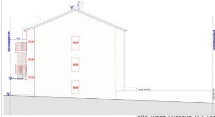
SÜD-WEST ANSICHT M 1:100
