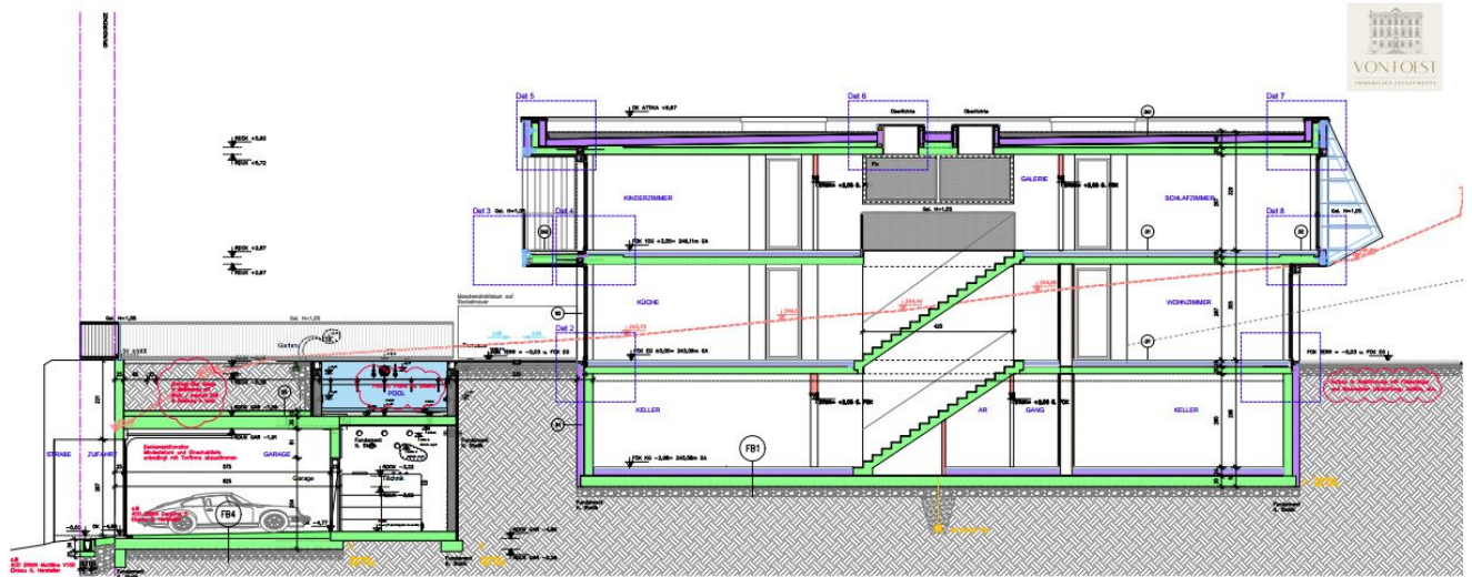
SCHNITT BB
