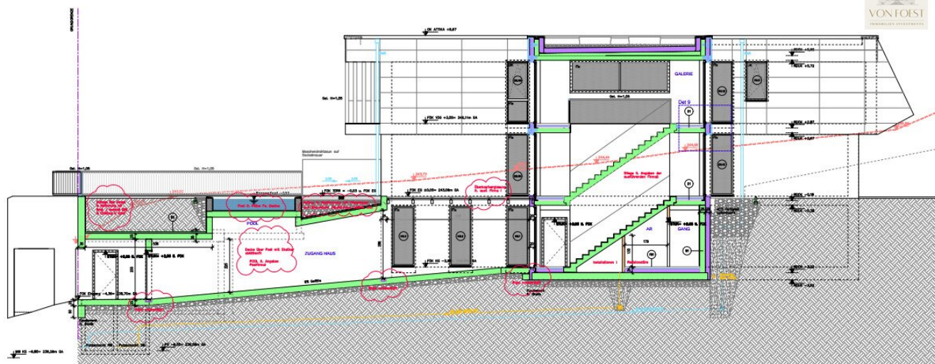
SCHNITT AA
