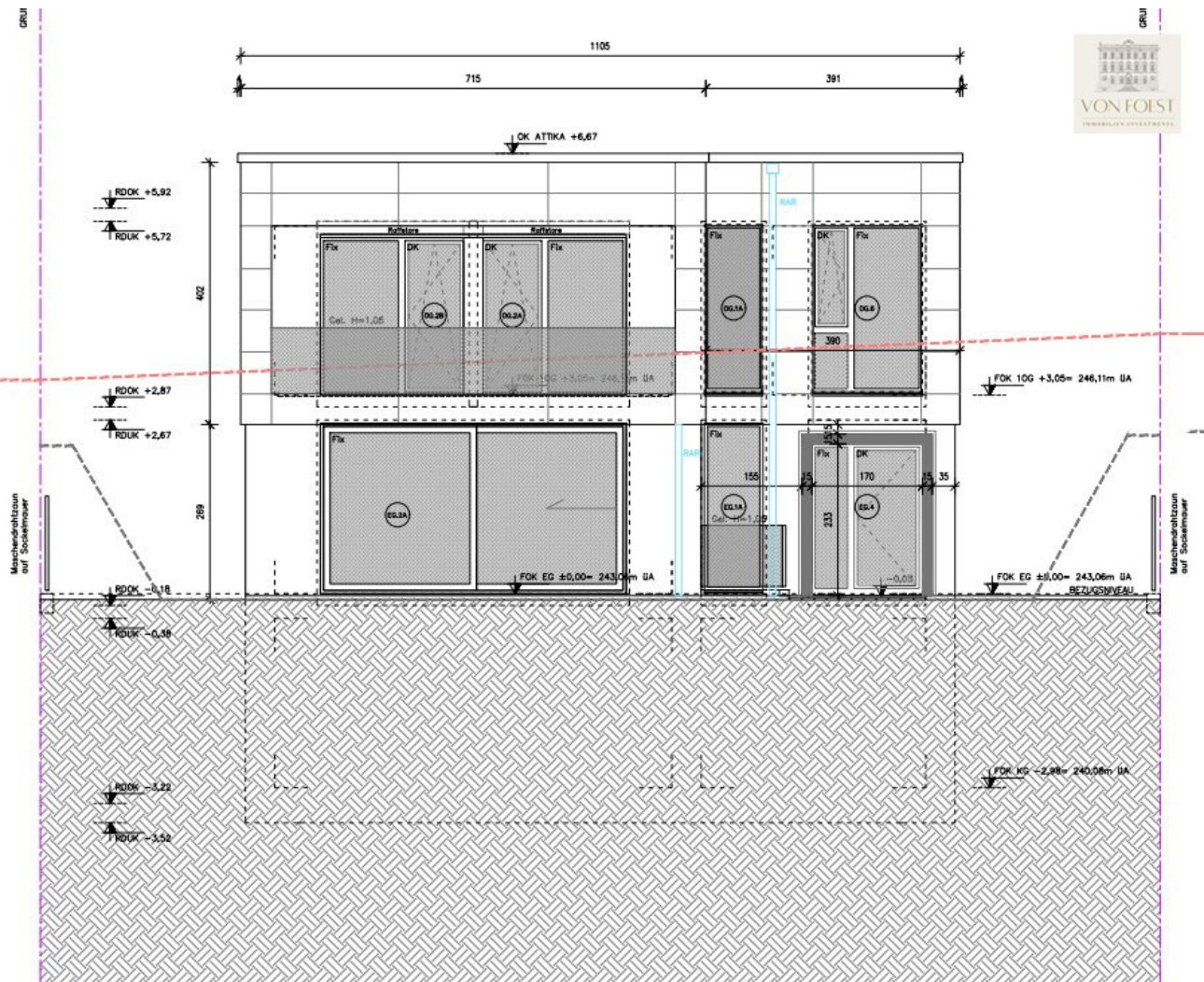
ANSICHT WEST
