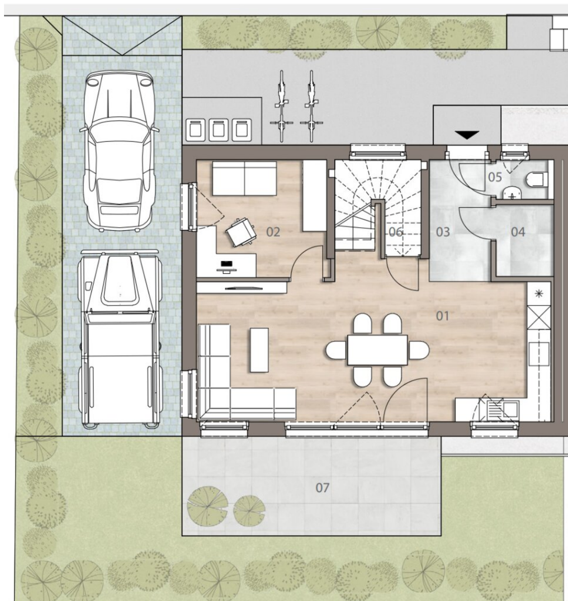
Erdgeschoss
