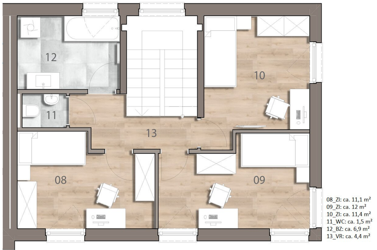
Obergeschoss
