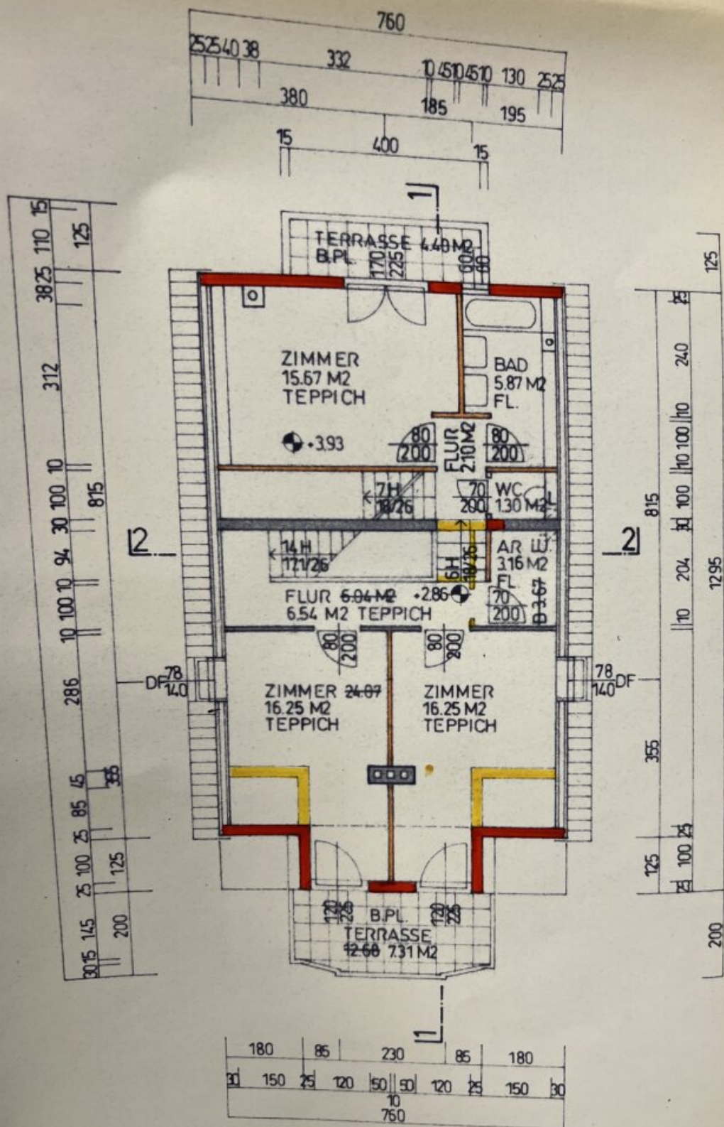
1. OBERGESCHOSS
