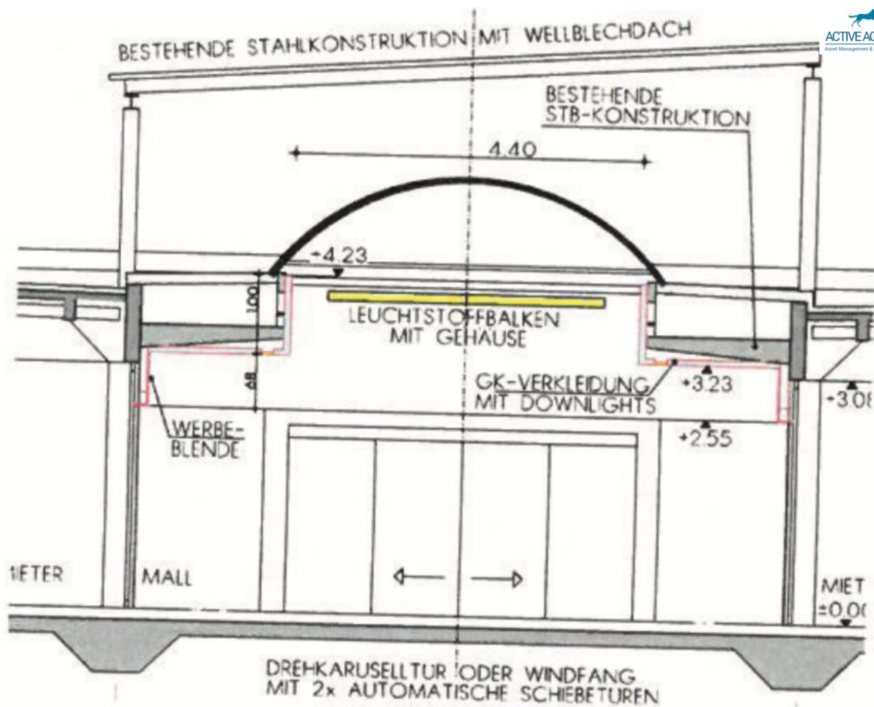
systemschnitt 1:50
