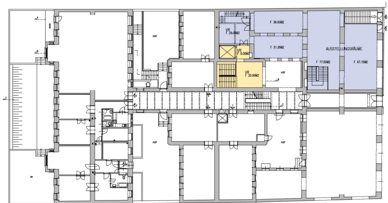
GRUNDRISS PARTERRE
