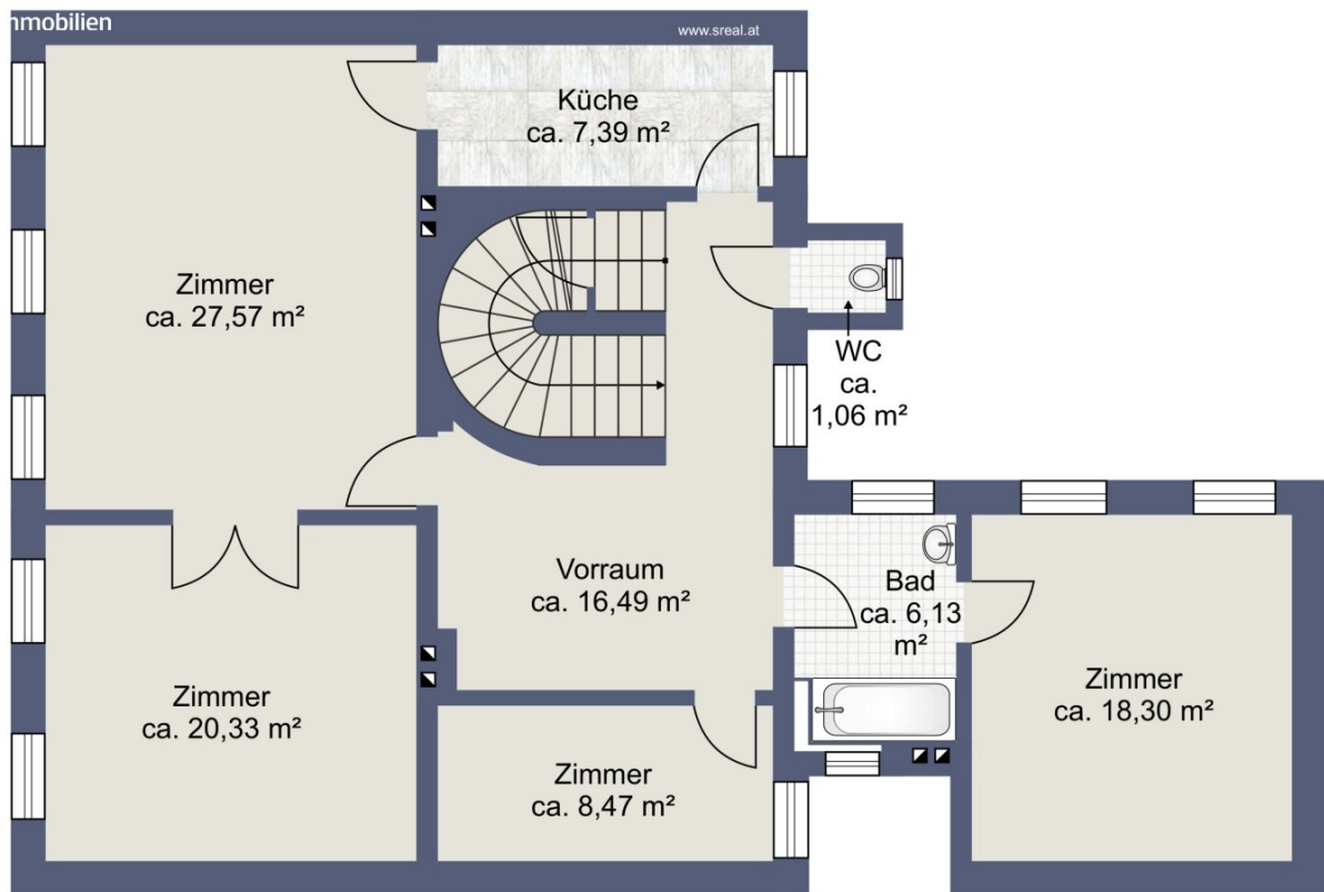
Skizze Obergeschoss
