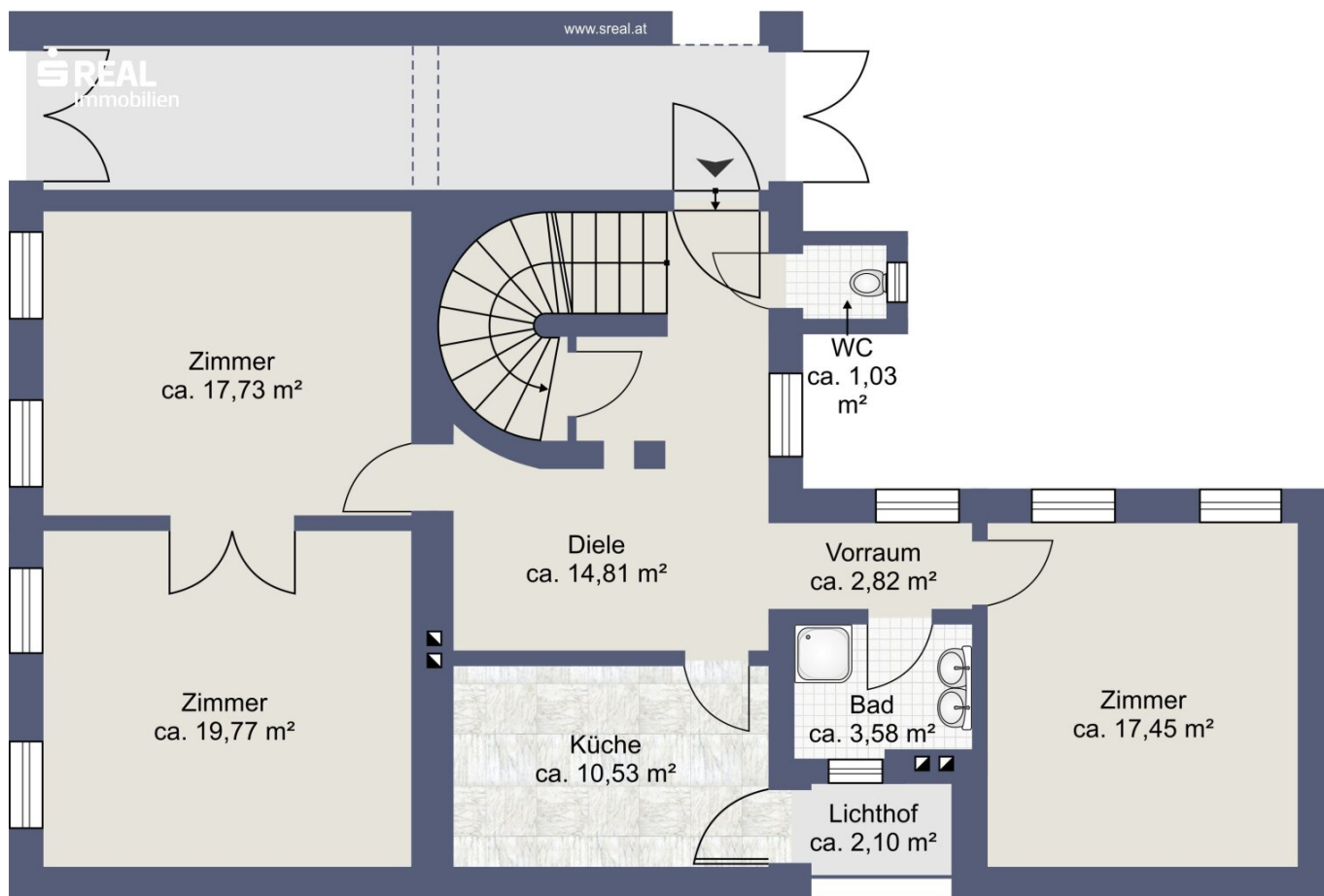
Skizze Erdgeschoss
