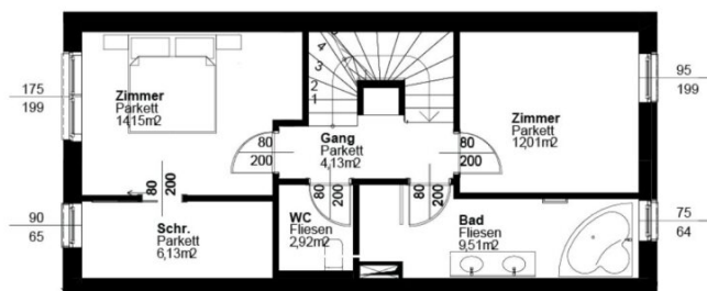
OG
