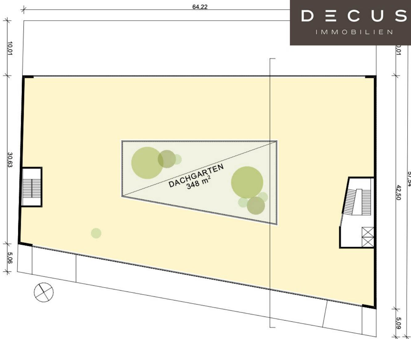
1./2. OG M 1:500
