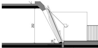
Schnitt 47.B
