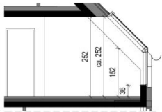
Schnitt 47.A
