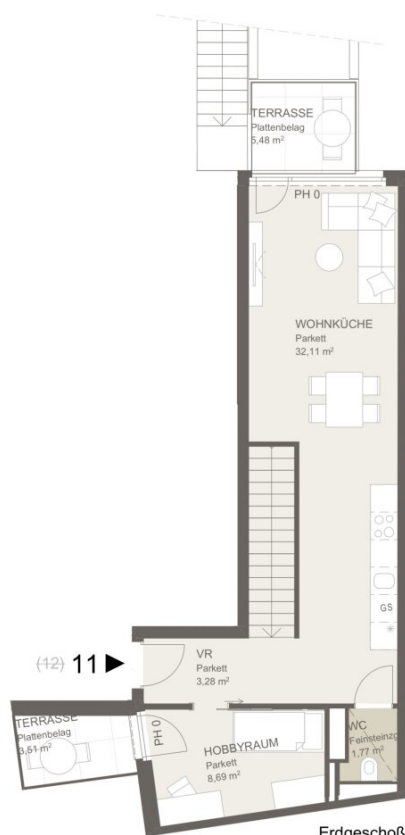
Erdgeschoß
