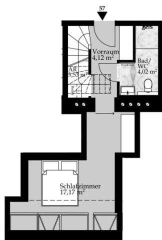
Dachgeschoss 1
