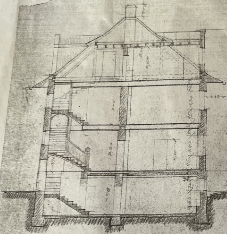
QUERSCHNITT
