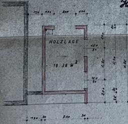
Untergeschoß
