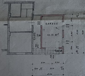
Erdgeschoß
