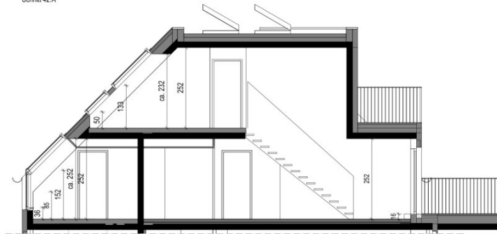
Schnitt 42.B
