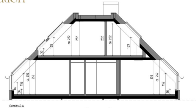
Schnitt 42.A
