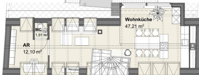
2. DACHGESCHOSS | TOP 7 | M 1:100
