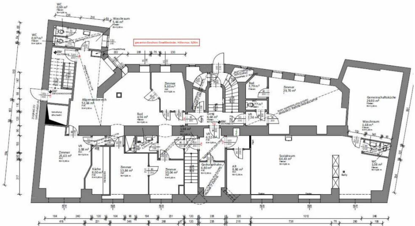
GRUNDRISS SOUTERRAIN
