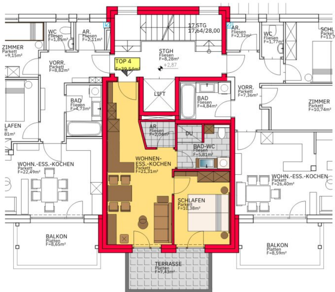
OBERGESCHOSS M 1:100
