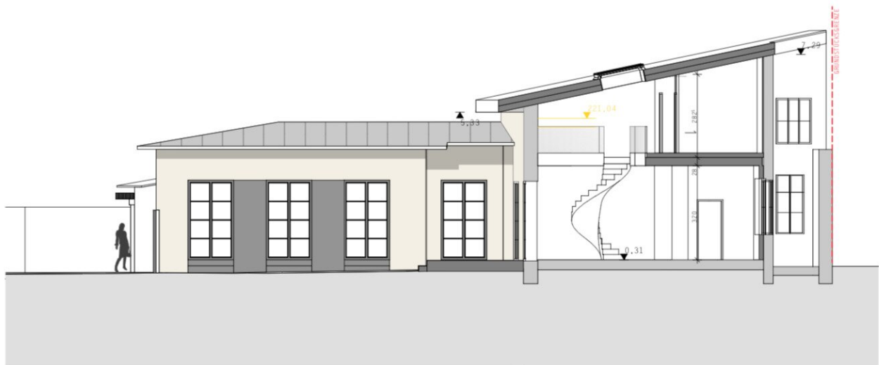
GARTENOBJEKT SCHNITT
