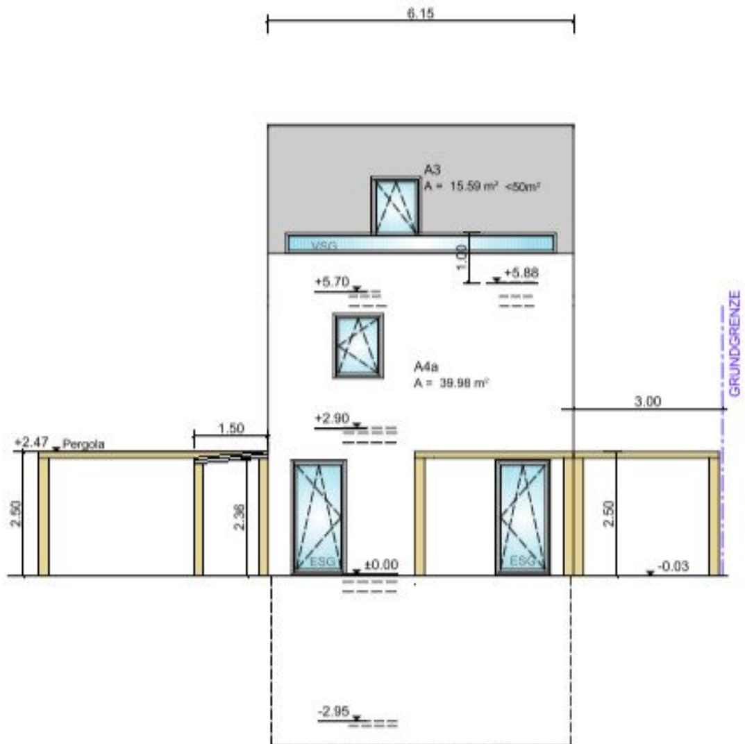
WEST - ANSICHT
