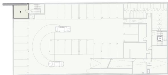
GRUNDRISS KG
