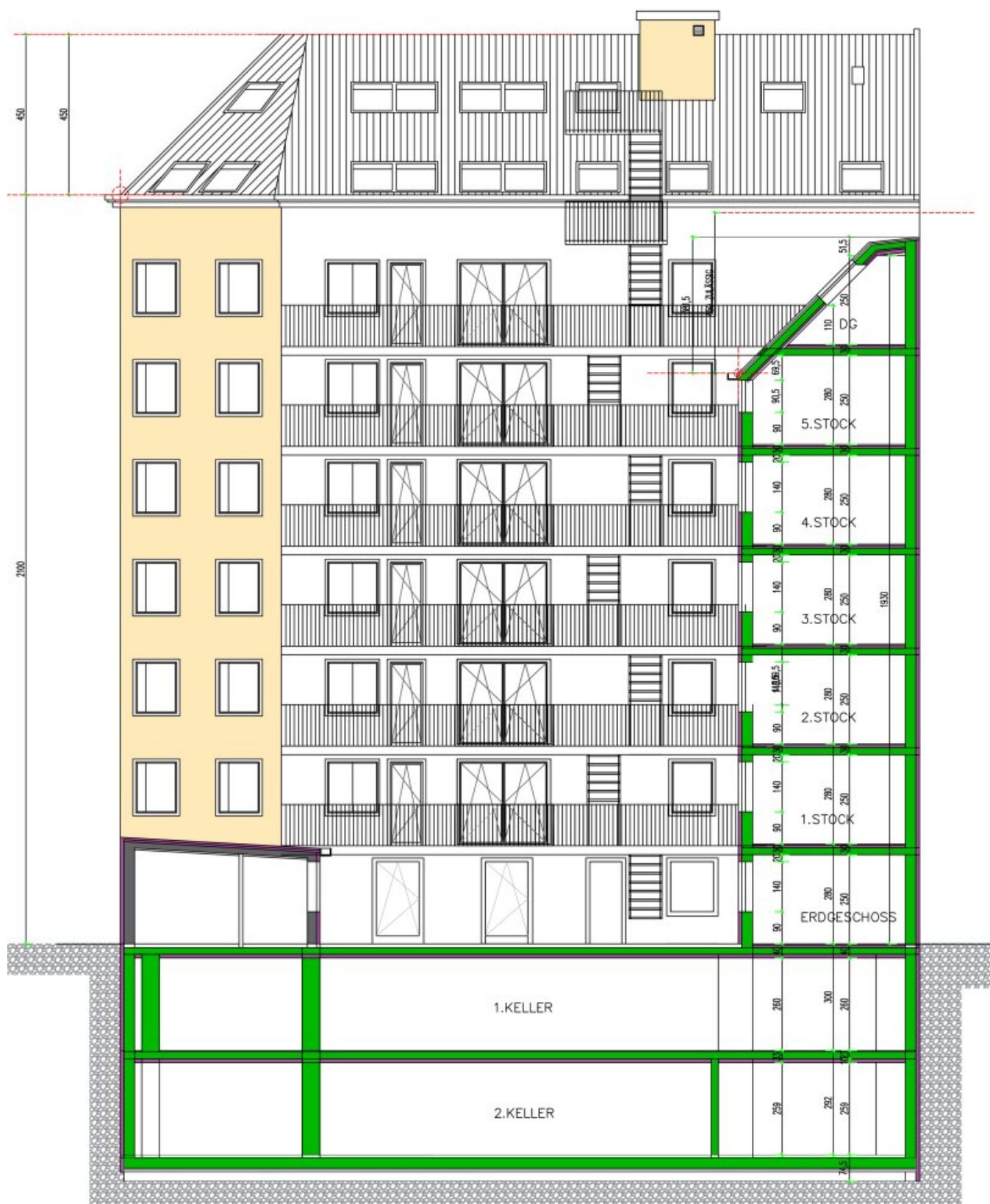
SCHNITT A-A
