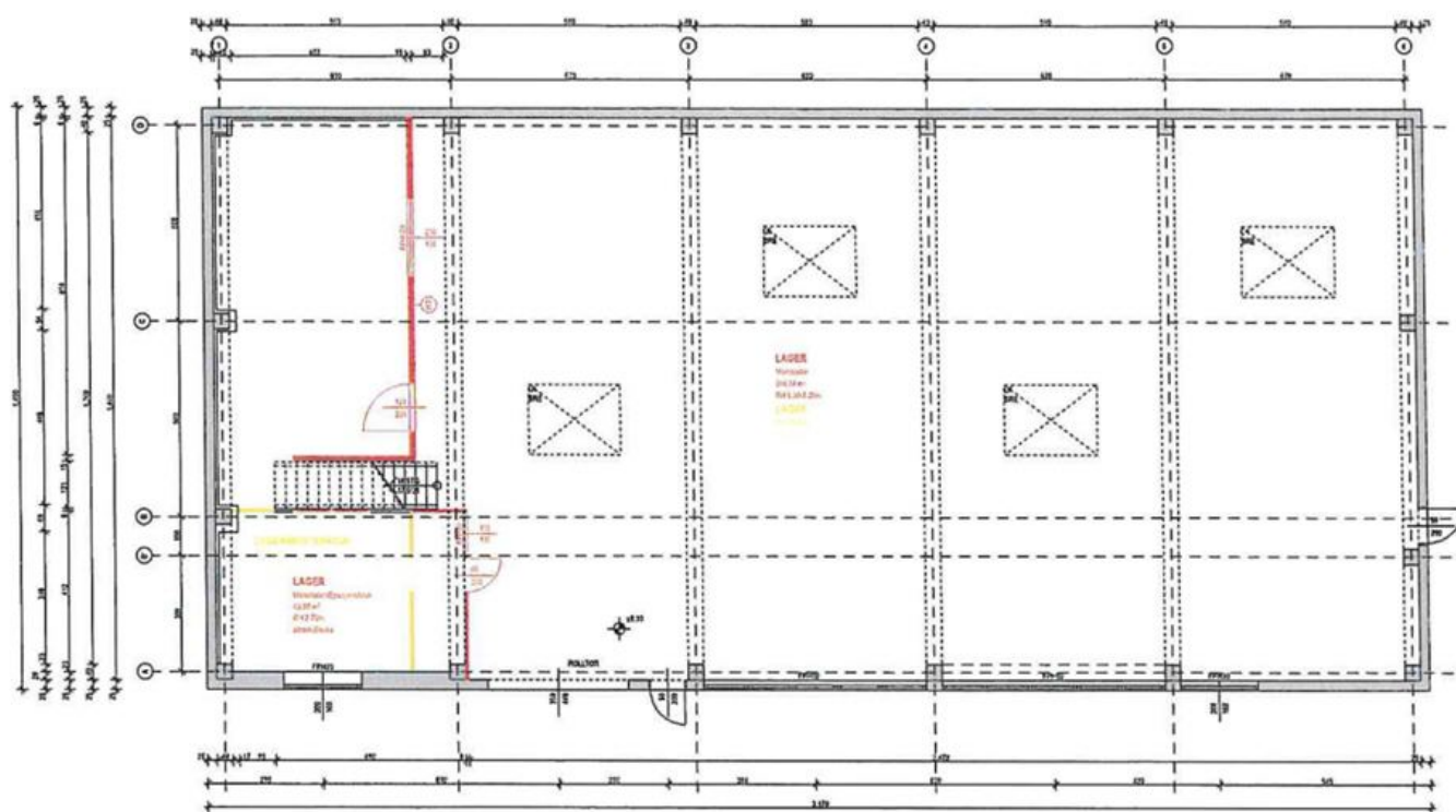
Lagerhalle EG 1:100
