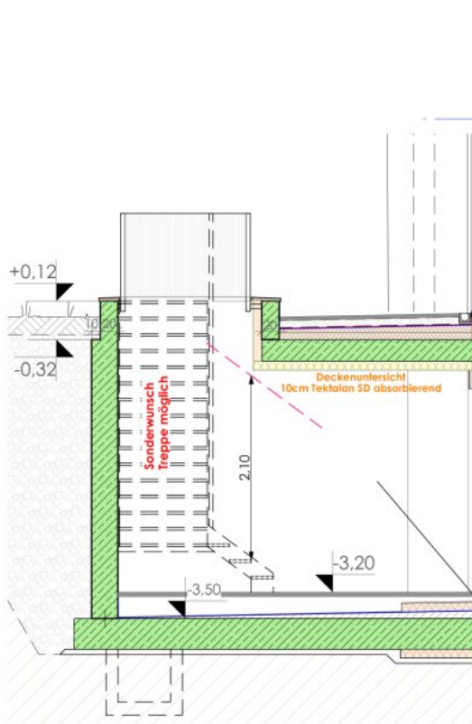
SNITT LICHTHOF
