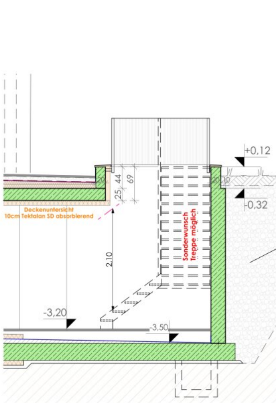
SCHNITT LICHTHOF
