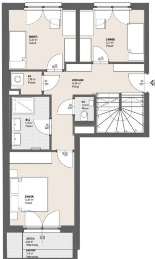
1. Dachgeschoß
