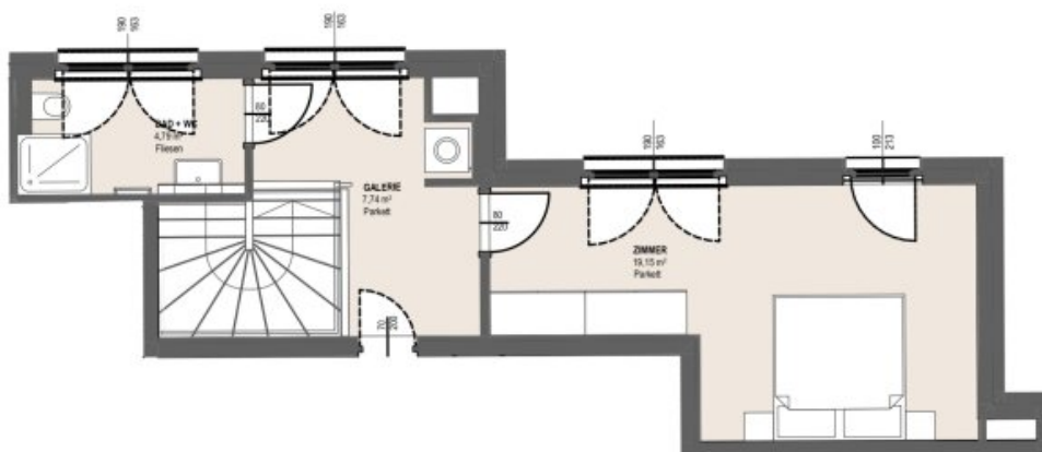
2. Dachgeschoß
