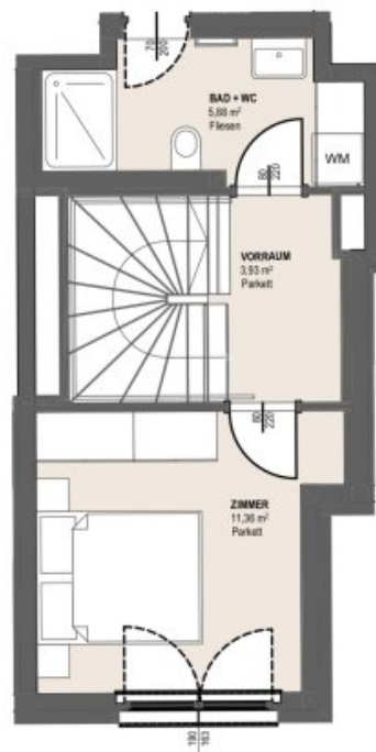
2. Dachgeschoß
