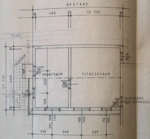
GRUNDRISS 1. OG
