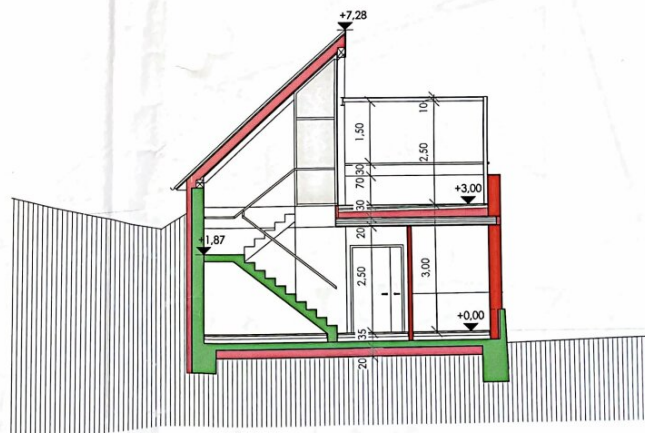
SCHNITT 2
