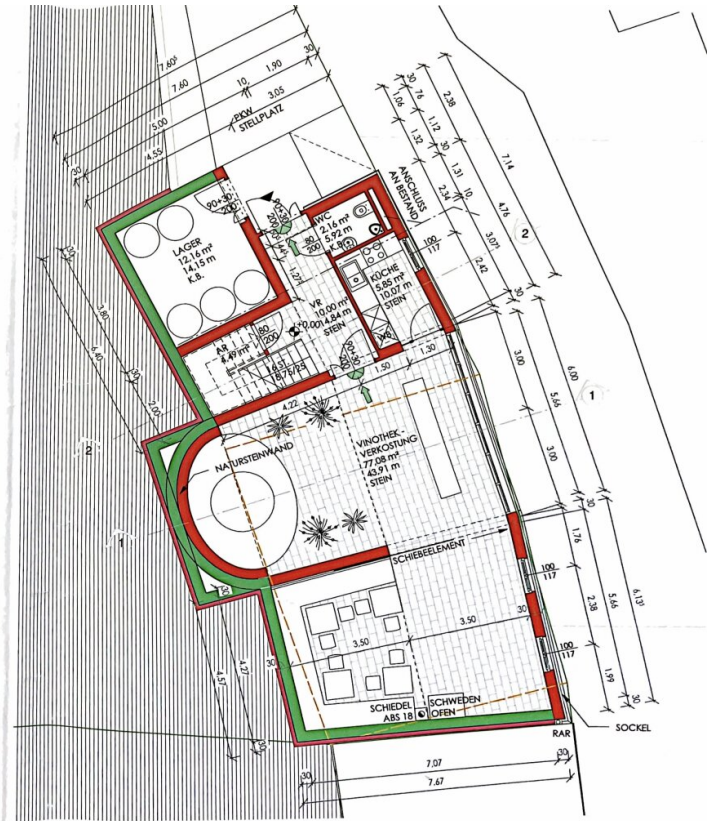
GRUNDRISS EG
