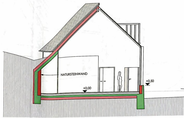
SCHNITT 1
