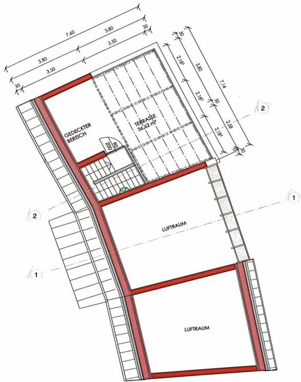
GRUNDRISS 1.OG
