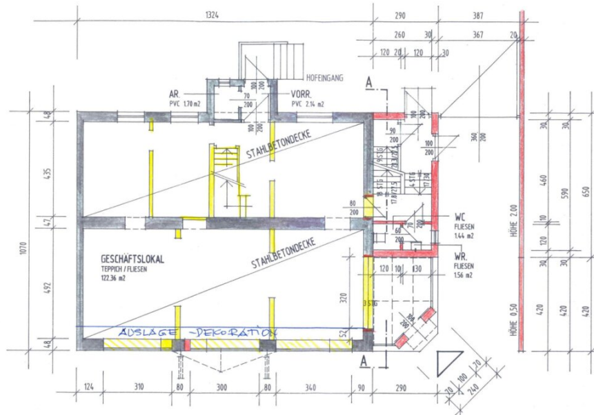
GRUNDRISS ERDGESCHOSS
