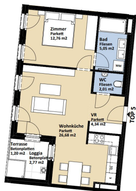
Grundriss TOP 5 Obergeschoß 1:100
