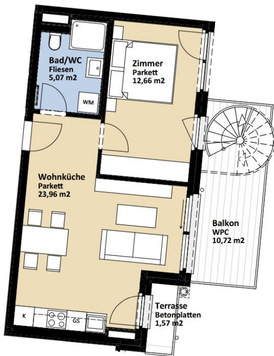
Grundriss TOP 11 Dachgeschoss 1:100
