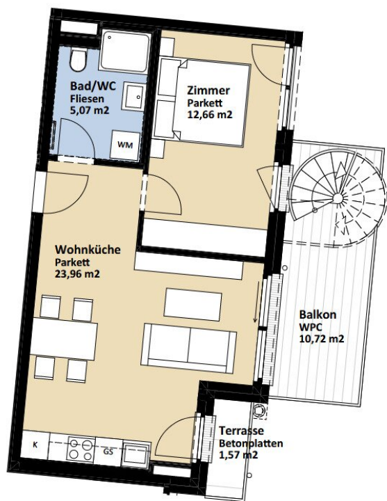
Grundriss TOP 11 Dachgeschoss 1:100
