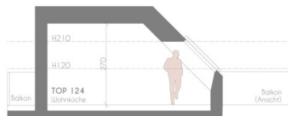
Schnitt I
