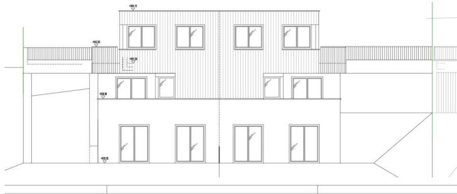
ANSICHT NORD
