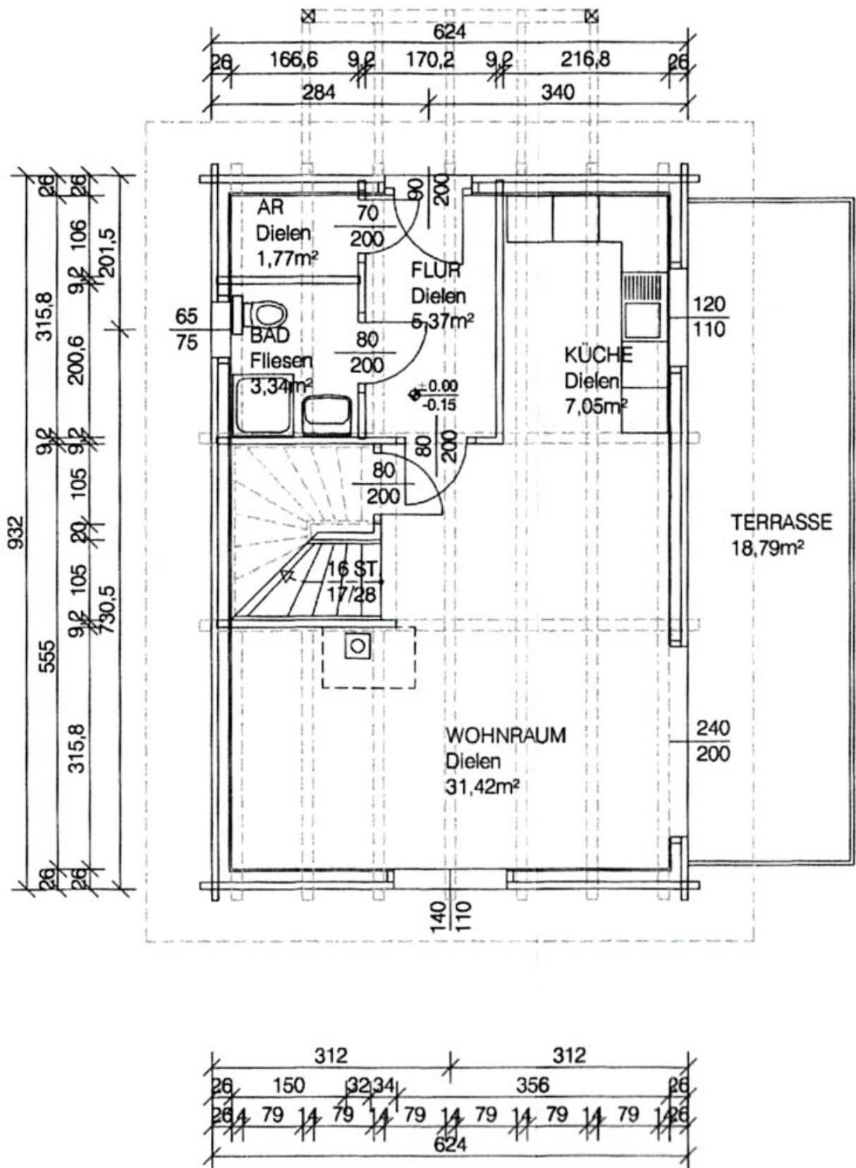
GRUNDRISS ERDGESCHOSS
