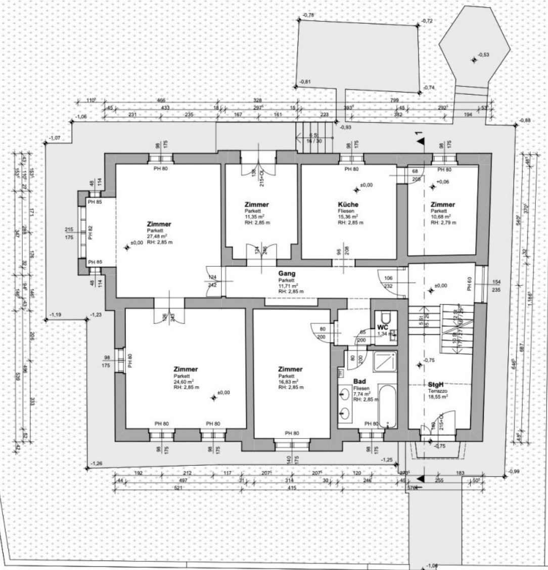
Erdgeschoss
