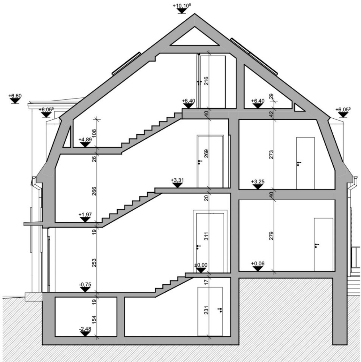
Schnitt 1-1
