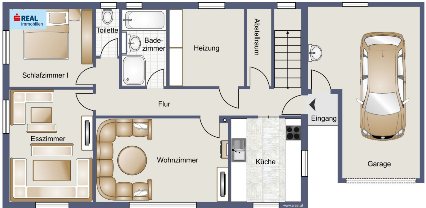
Skizze Erdgeschoss
