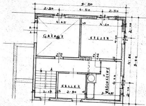
MESEEGRUNDRISS
