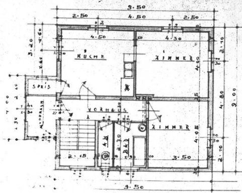
PARTEREGRUNDRISS
